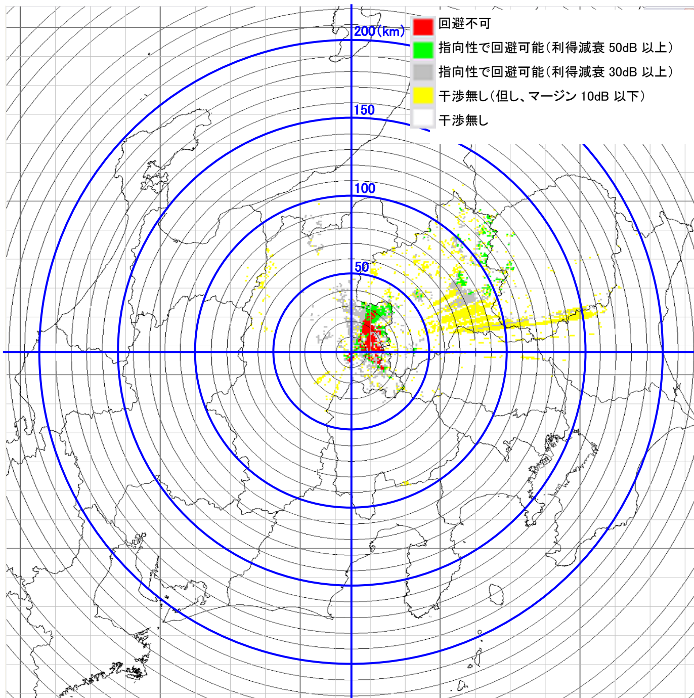
12-① JAXA 臼田電界強度マップ・・・φ60cm パラボラアンテナ送信機
