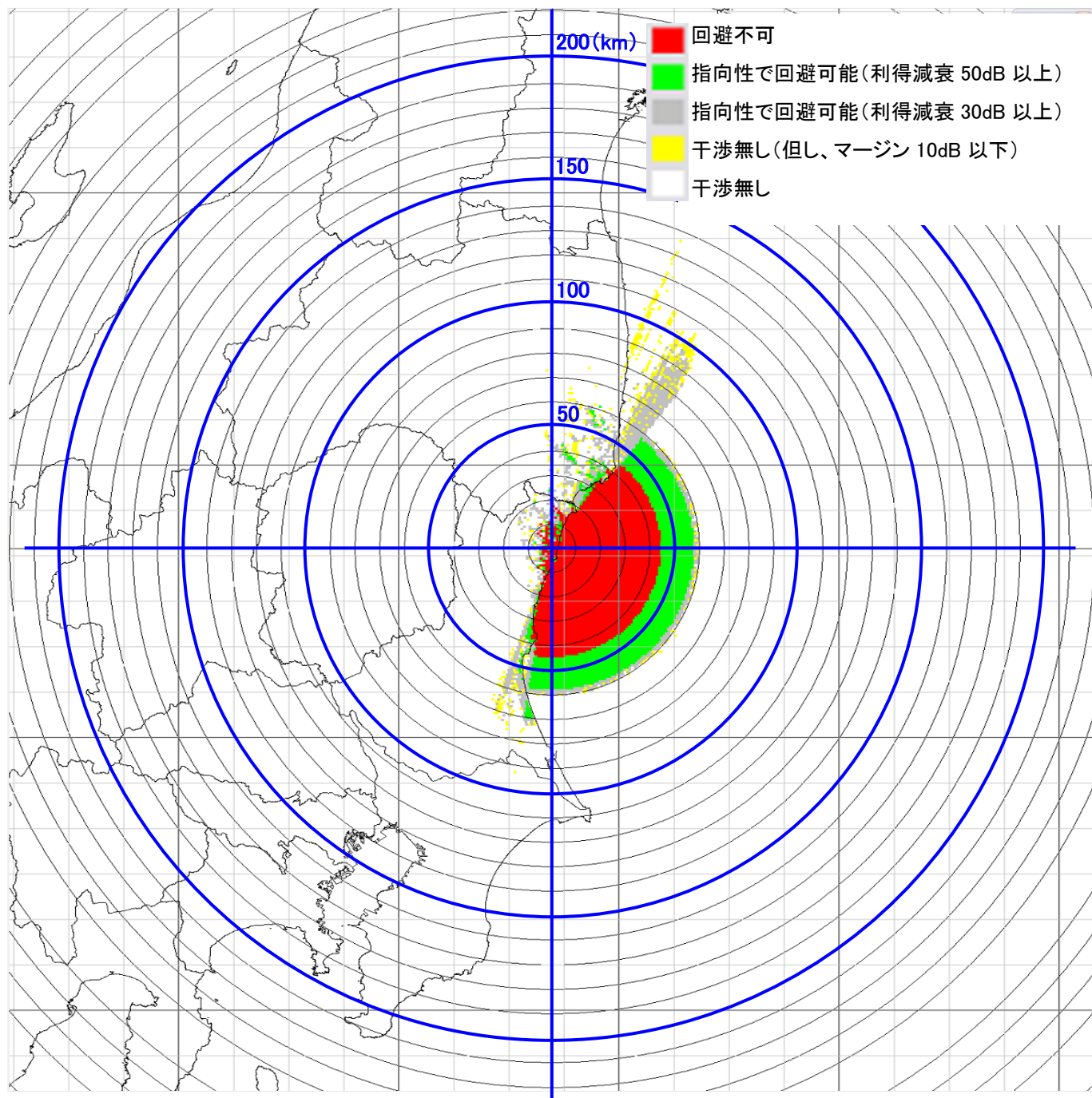
8-① 日立 電界強度マップ・・・φ60cm パラボラアンテナ送信機
