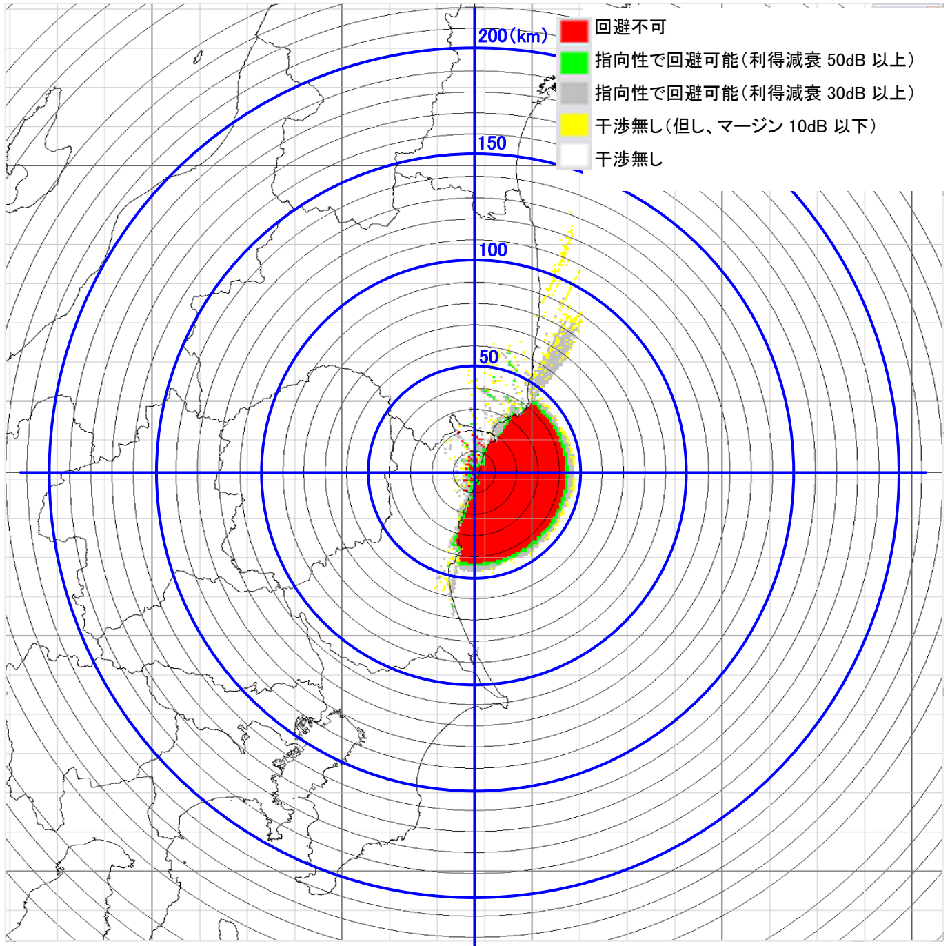
7-① 高萩 電界強度マップ・・・φ60cm パラボラアンテナ送信機
